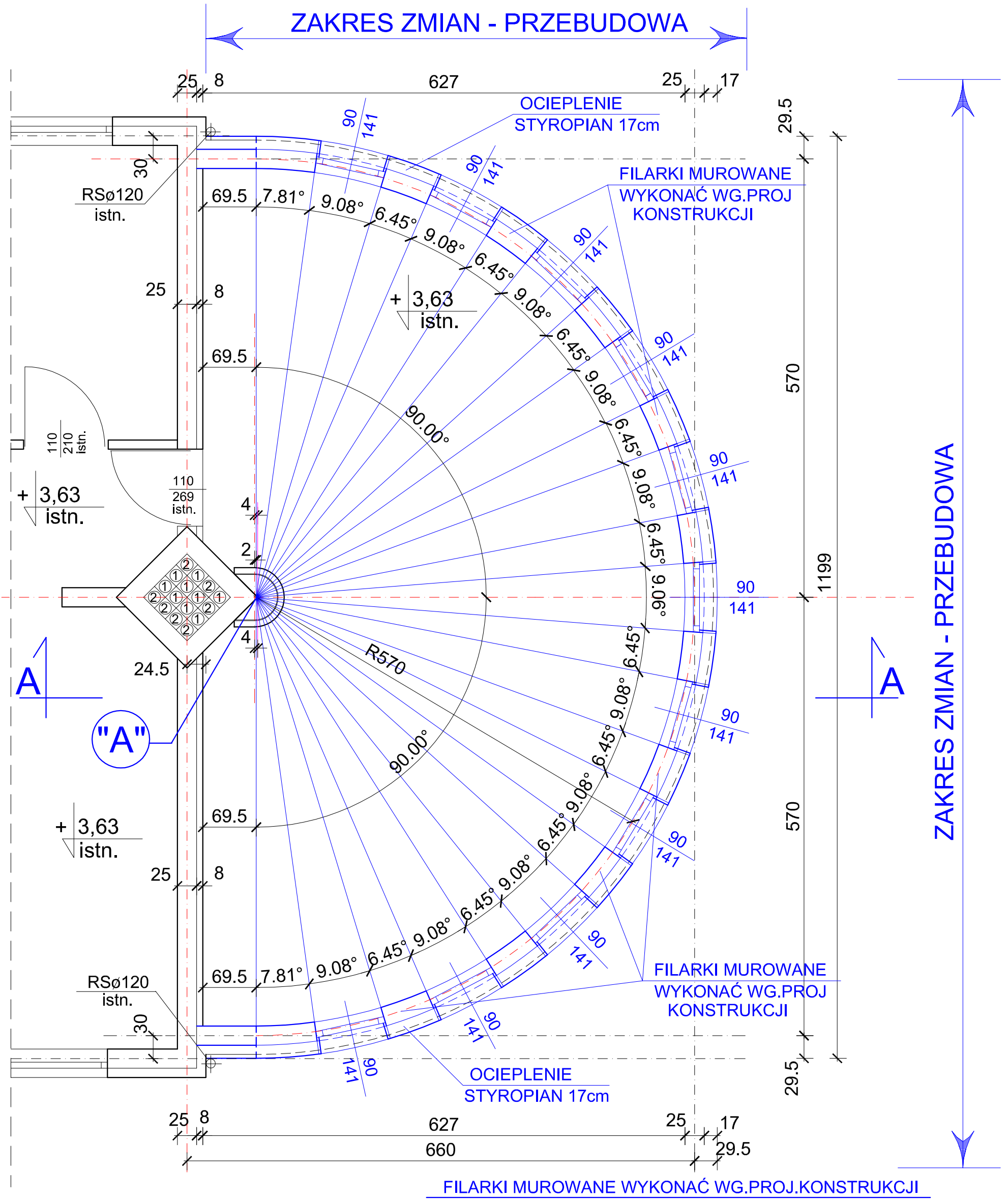
"A" - PUNKT BAZOWY PRZY TYCZENIU FILARKÓW I OKIEN ORAZ OKAPU
